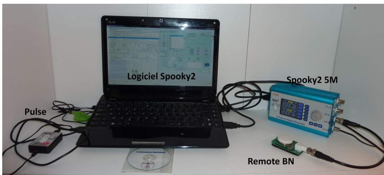
CONFIGURATION REMOTE BN. A DISTANCE AVEC LES ONDES SCALAIRES.
